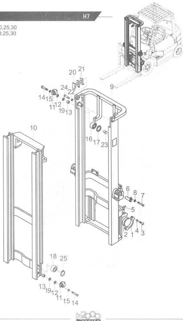
门架(基本型)/MAST (NORMAL MAST M)
