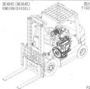
发动机(柴油机) ENGIEN (DIESEL)
