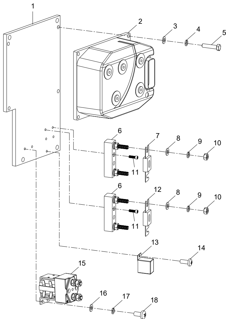
图 16 电气系统 II Fig.16 Electrical system II
