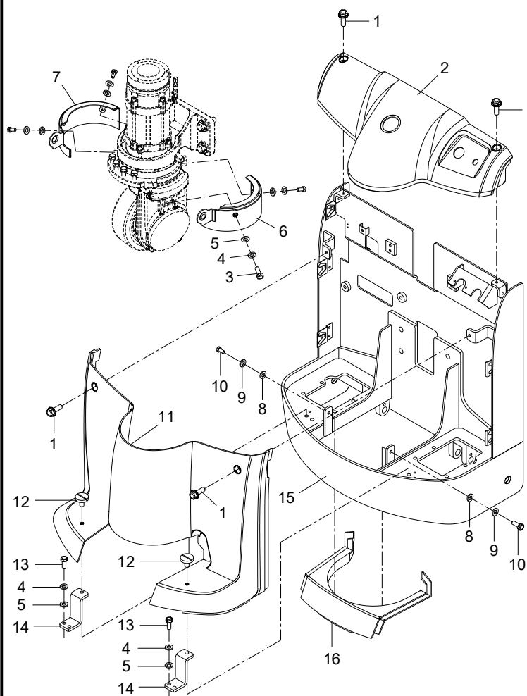
图 11 车身系统 II Fig.11 Body system II
