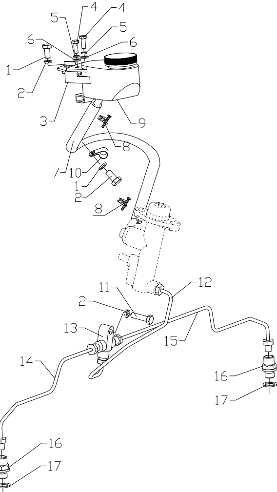
图9 管路总成 Fig.9 Brake pipe assey
