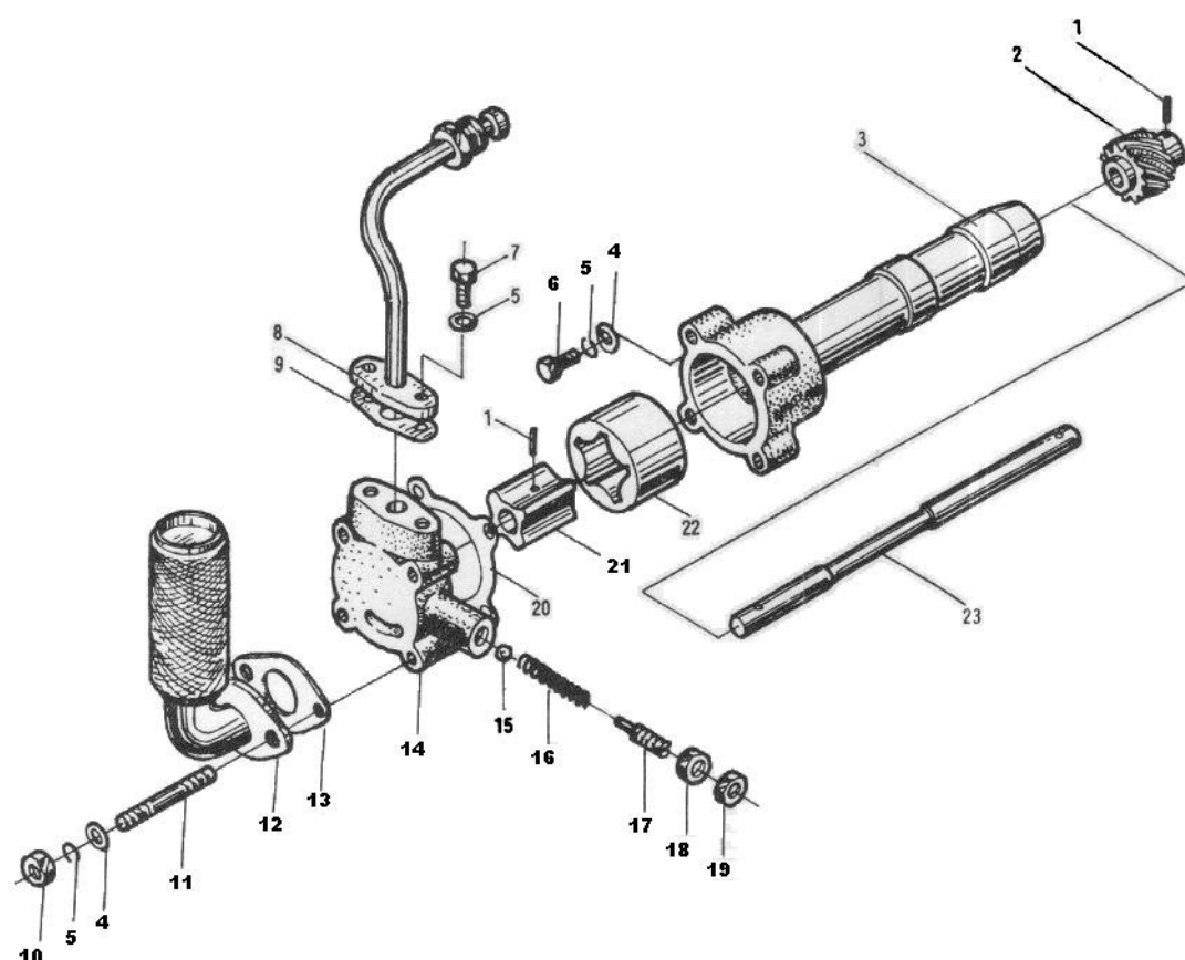
Масляный насос и маслопровод в сборе
