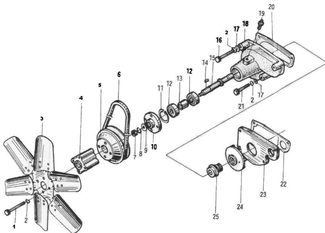
РИС. 9 Система охлаждения, водяная помпа и вентилятор в сборе
