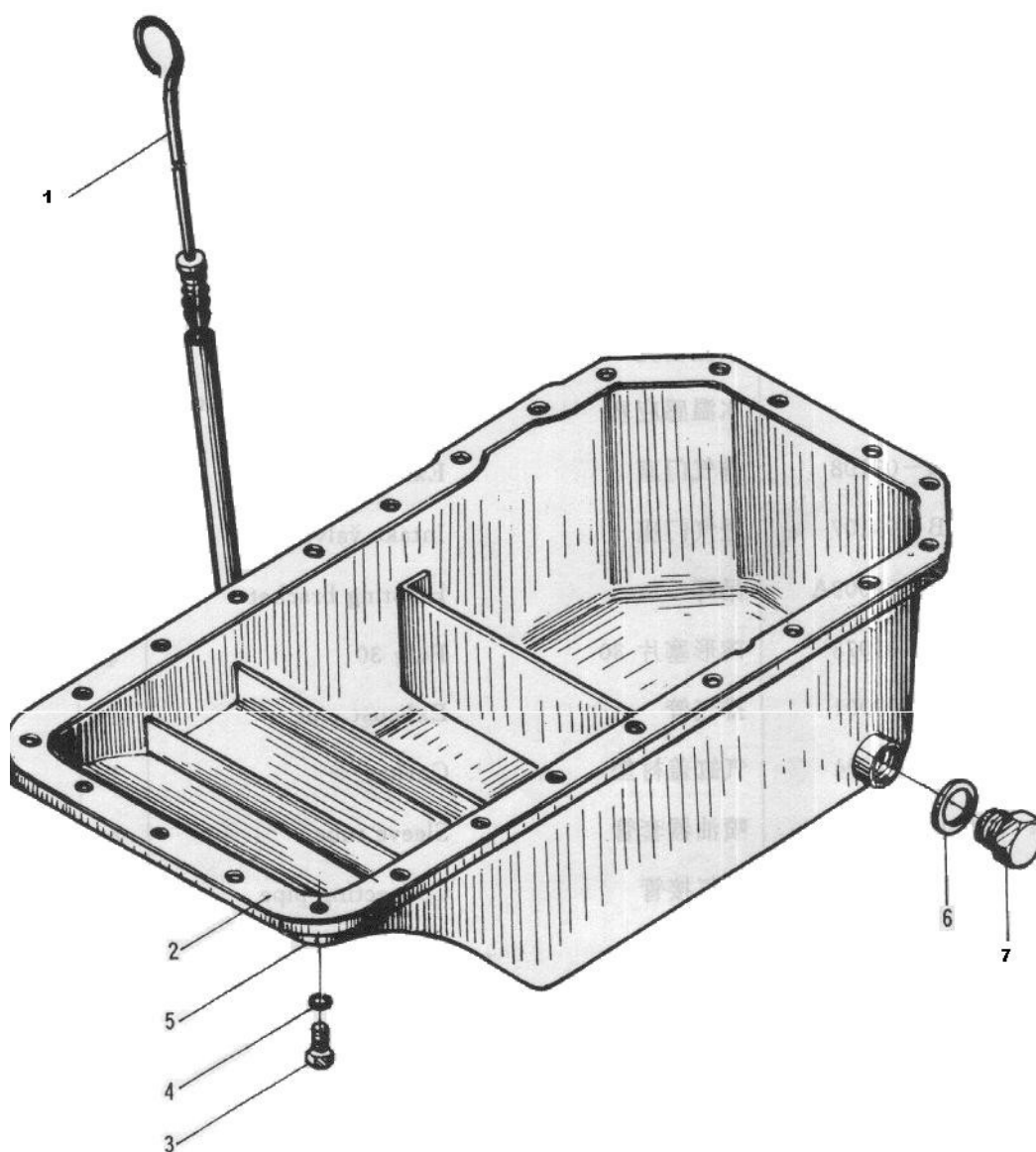
РИС. 3 Картер двигателя в сборе
