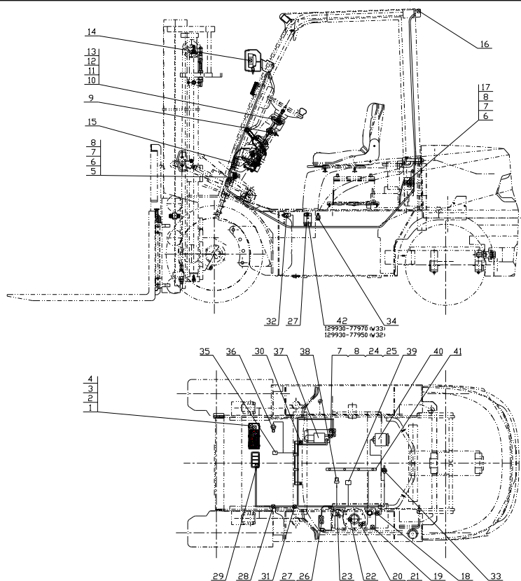
图5 电气系统 Fig.5 Electrical system
