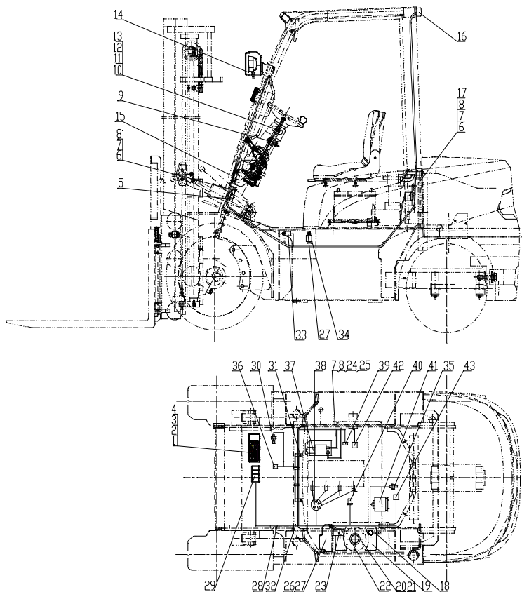
图2 电气系统 Fig.2 Electrical system
